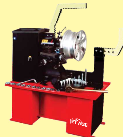
Alloy Rim Straightener
